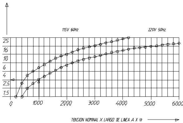
SECCION DE LA LINEA EN mm 2
